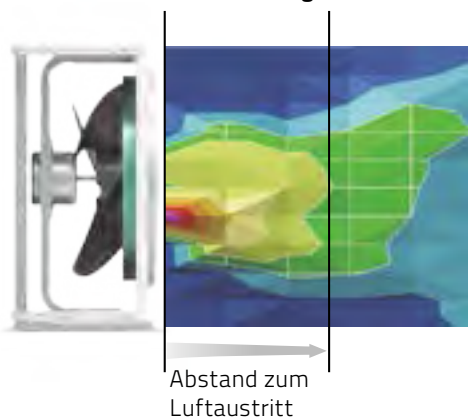
Herkömmliche Luftführung
